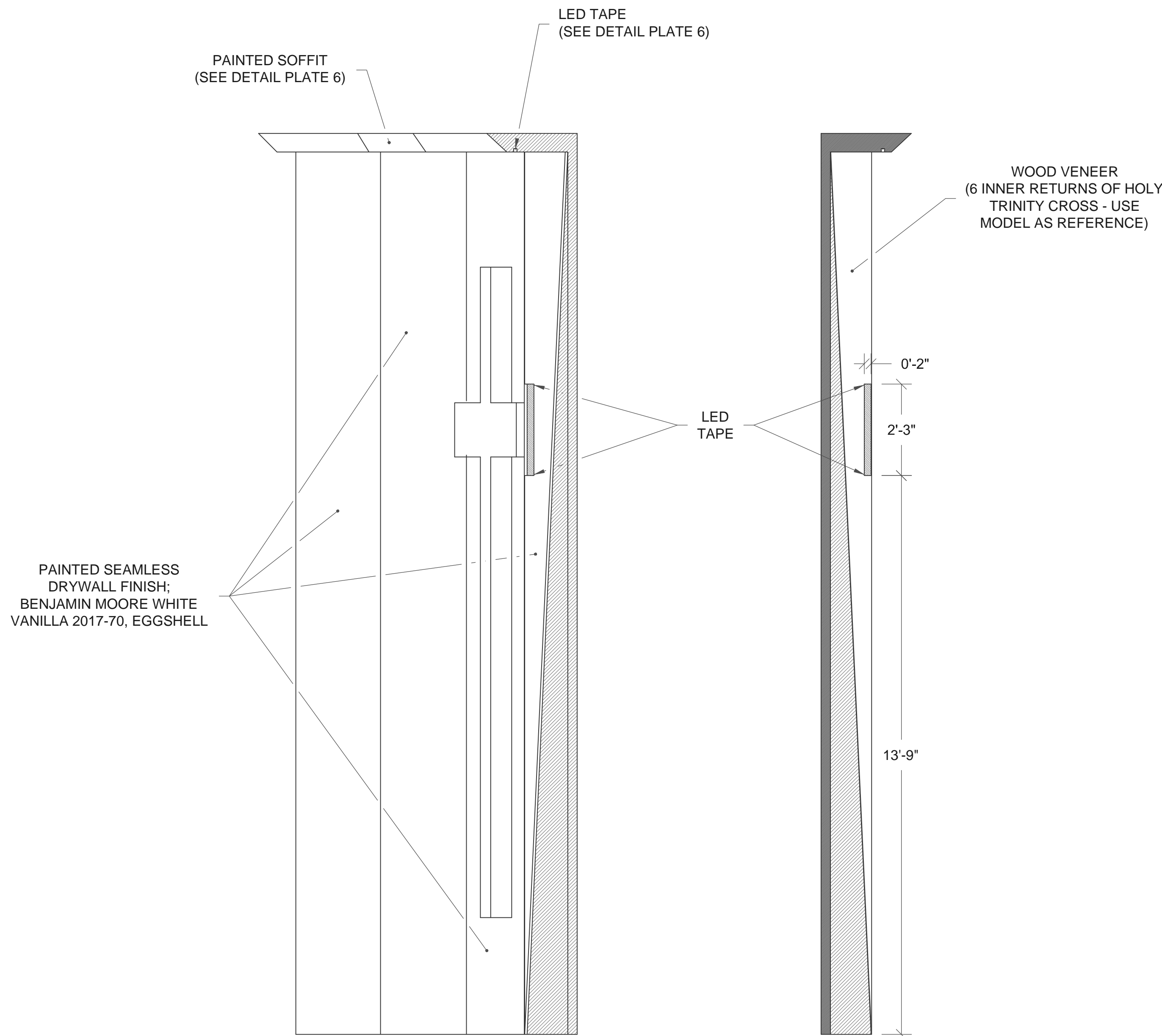
SECTION B:B'
