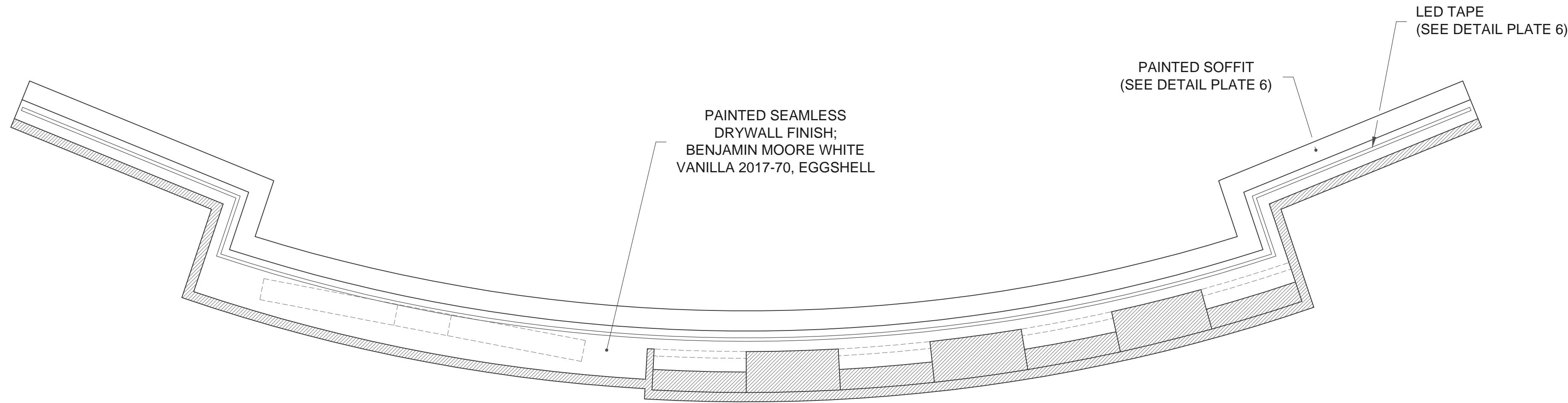
SECTION A:A' | SOFFIT
